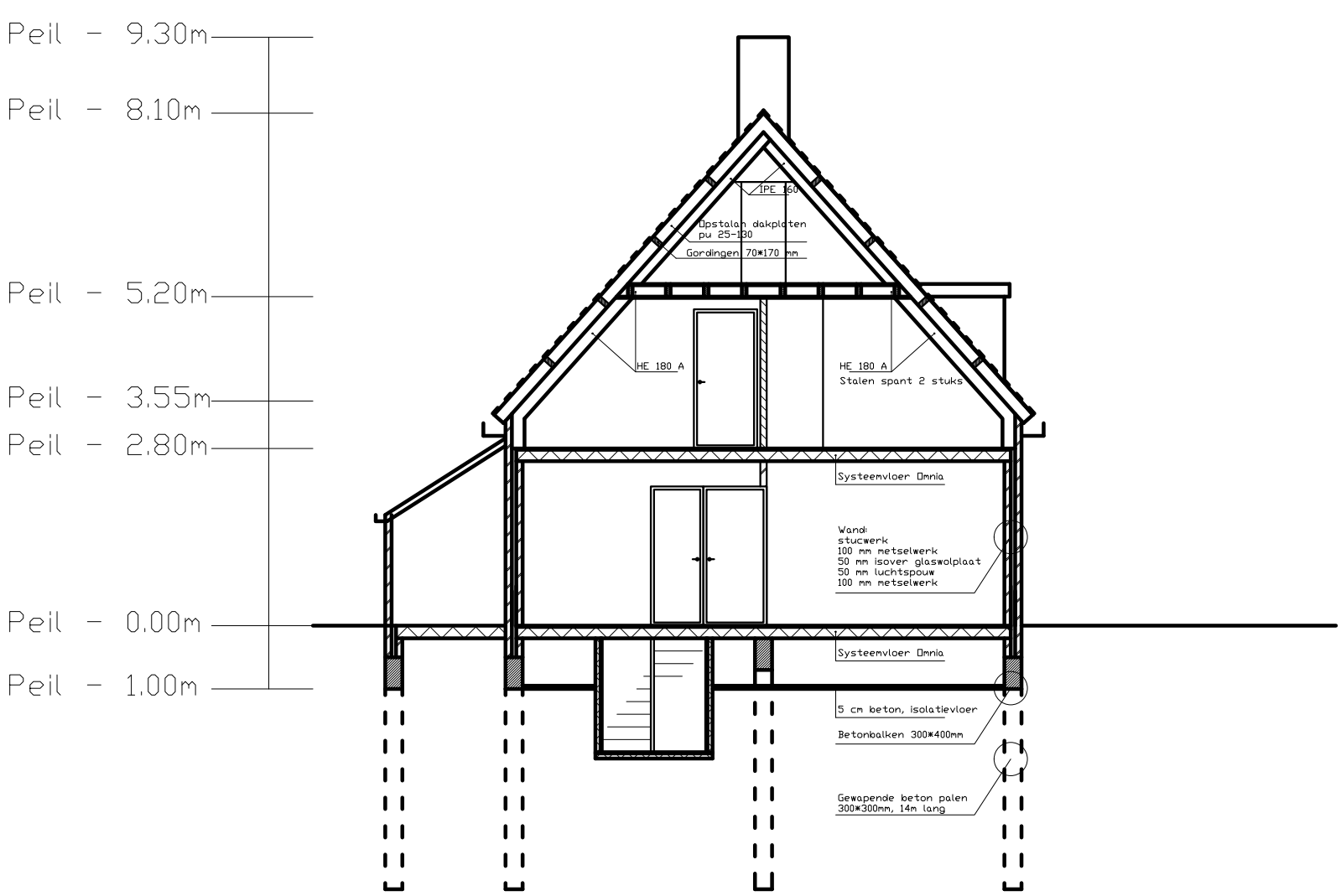
doorsnede A-A zuidgevel
