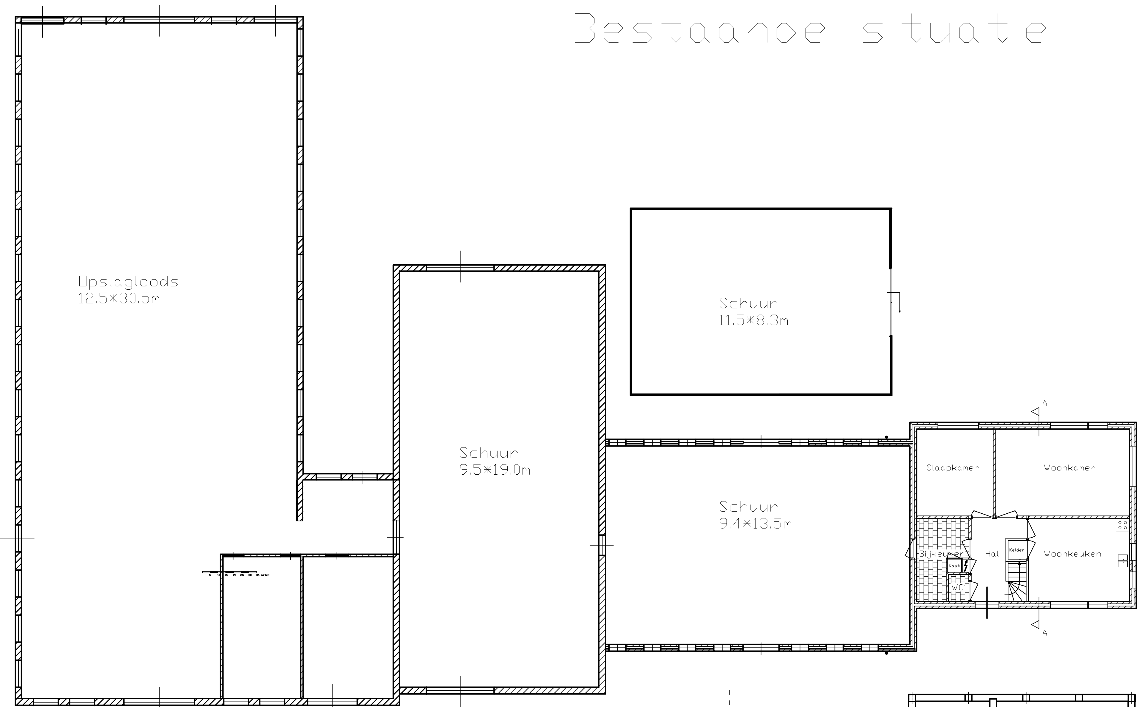
Plattegrond
