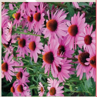
2 Echinacea purpurea 'Magnus'
