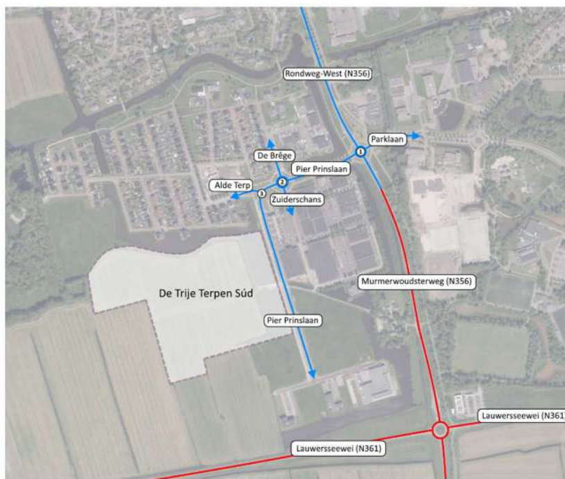
Figuur 2.1 Huidige verkeersstructuur nabij het plangebied
