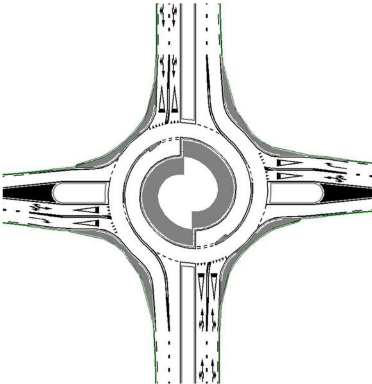
Figuur 5.1 Turborotonde voorbeeld (Meerstrooksrotondeverkenner)
