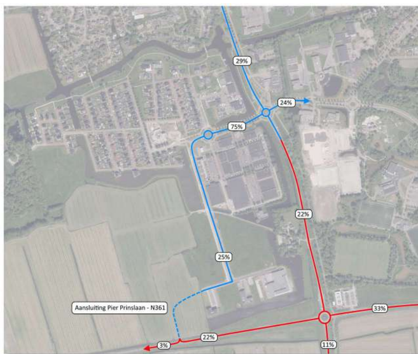
Figuur 5.1 Verkeersstromen aansluiting N361
