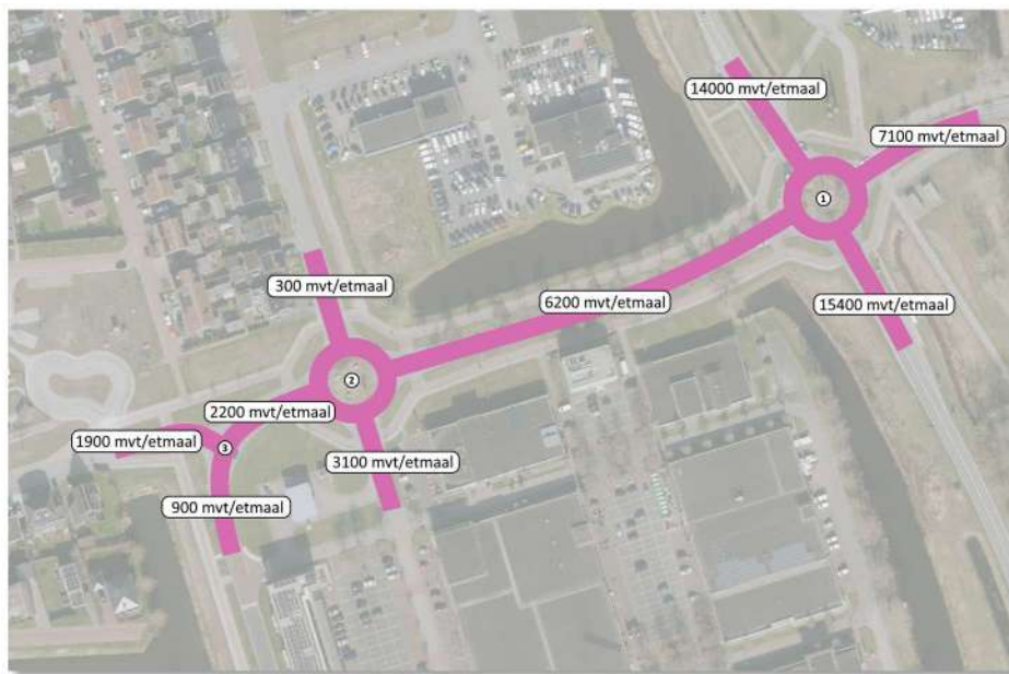
Figuur 4.1 Toekomstige intensiteiten scenario 1
