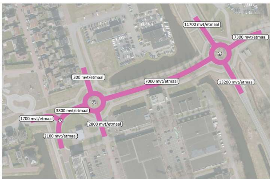
Figuur 4.2 Toekomstige intensiteiten scenario 2
