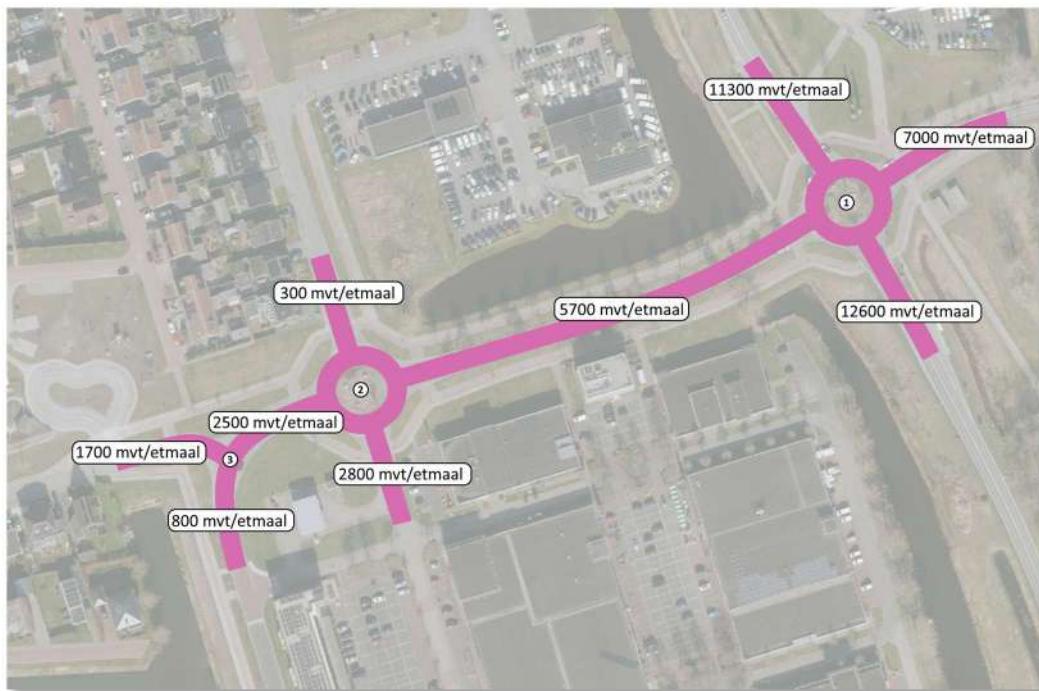
Figuur 2.4 Uitgebreid overzicht huidige werkdag intensiteiten
