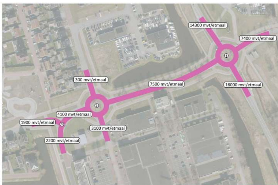
Figuur 4.3 Toekomstige intensiteiten scenario 3
