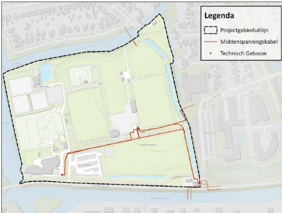
Figuur 18 Middenspanningskabel onder plangebied (bron: Antea)
