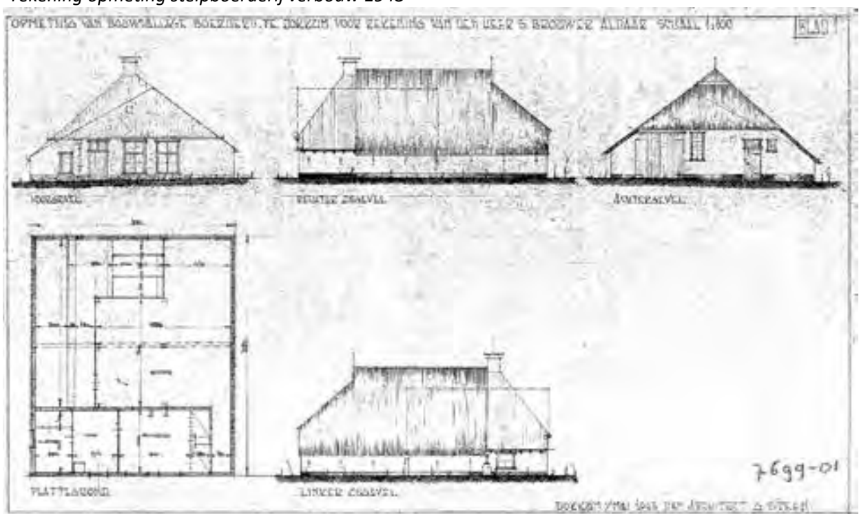
Tekening opmeting stelpboerderij verbouw 1943
