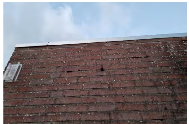
Figuren 11 en 12: Links, zicht op het gebouw van de tennisvereniging. Rechts, gedichte spouwvoegen en exclusion flaps op de muur.
