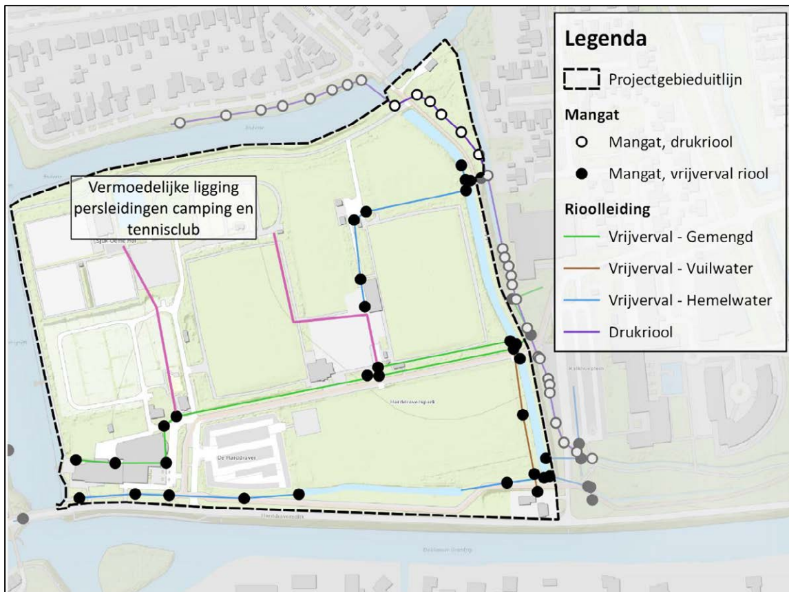
Figuur 3-2: Bestaand rioleringsysteem Harddraverspark (KLIC-melding 02-04-2024. Geverifieerd aan de hand van prints uit beheersysteem en riooltekeningen).
