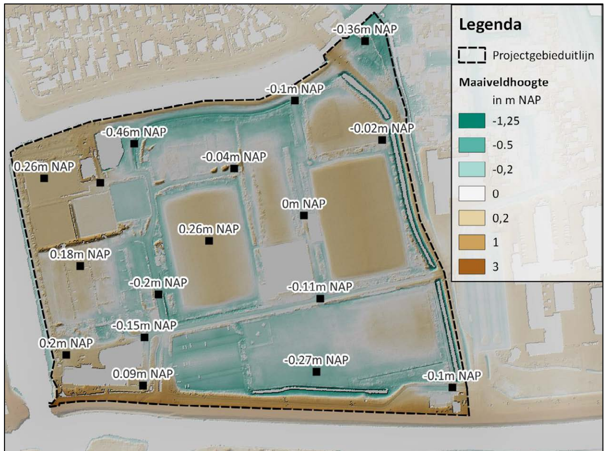
Figuur 3-3: Hoogtekaart van plangebied. Gebouwen aangeven in grijs (AHN4 DTM & BGT).
